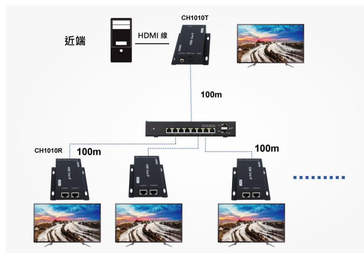
應用三：點對多點搭配Giga Switch延長+分配 不同區域顯示
