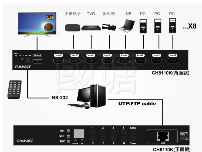
連接示意圖
